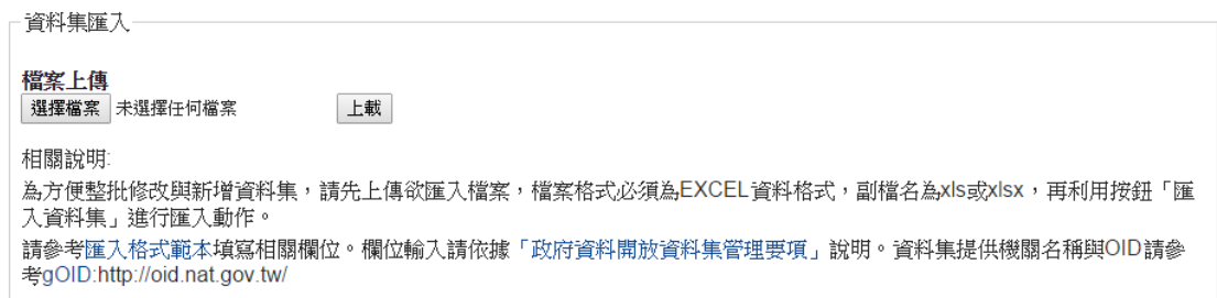
【圖 36】檔案上傳
